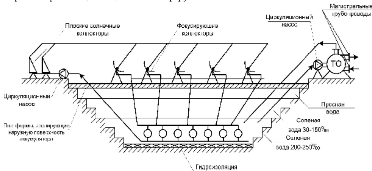
Рис. 3. Общая схема сезонного аккумулятора теплоты в пространстве отработанного карьера
