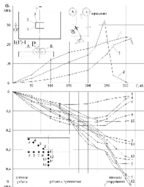
Рис.1. Зависимость напряжений в сжатой зоне бетона плиты и нормальных контактных напряжений под подошвой фундамента Φ-1-4 от уровня внешней нагрузки
