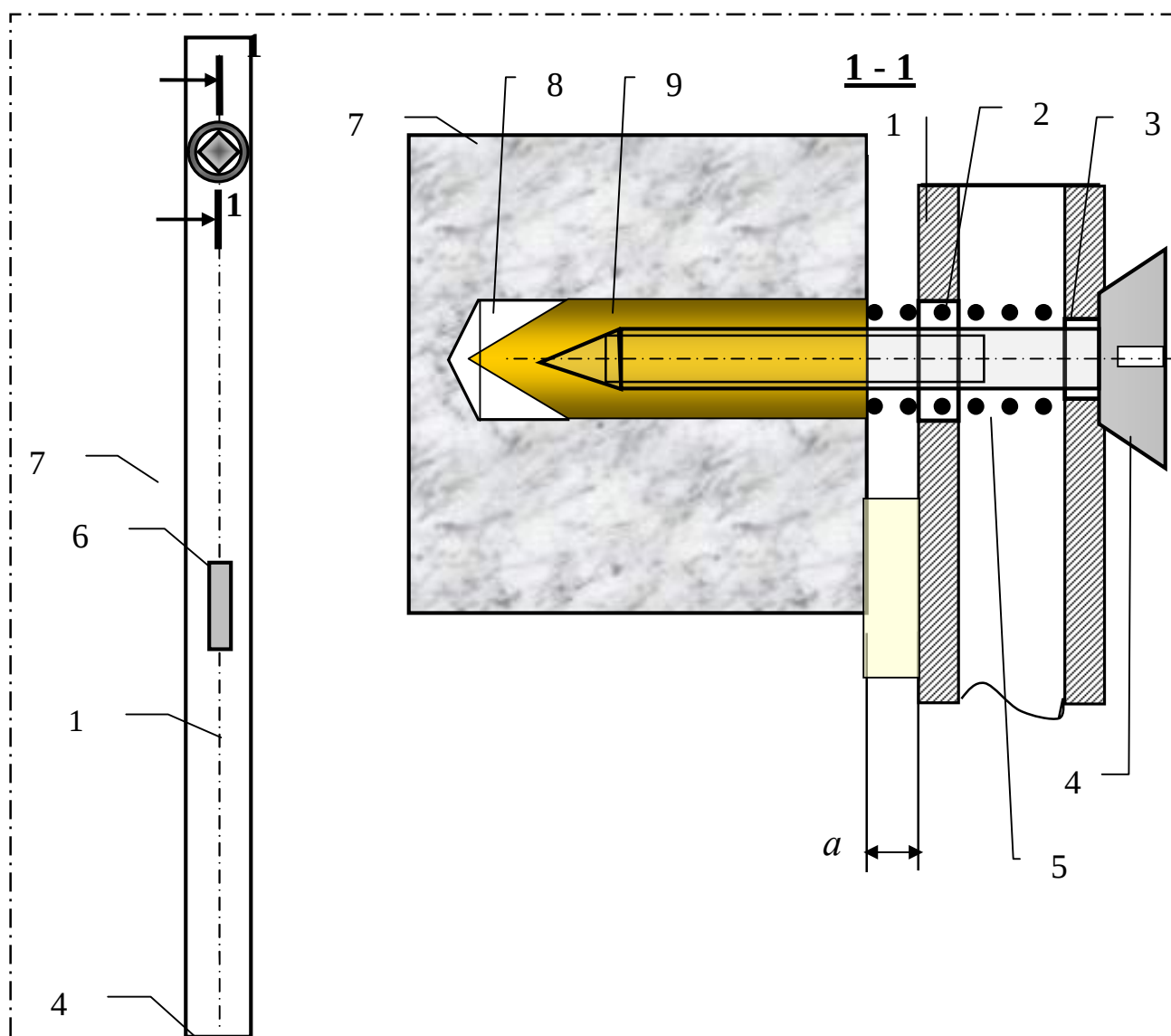
Рис. 1. Предложенная конструкция маячно-штукатурного уровня а) общий вид, б) разрез и способ установки
