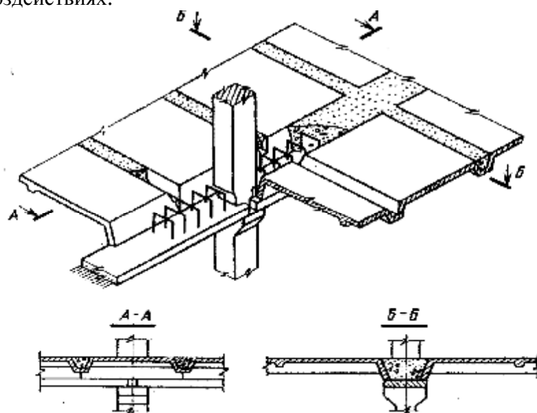
Рис. 2. Ребристые сборно-монолитные перекрытия с остовом из железобетонных панелей
