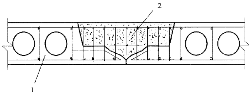
Рис. 5. Сборно-монолитное перекрытие:
