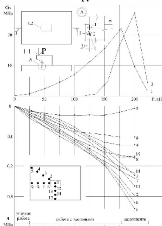
Рис.1. Зависимость напряжений в сжатой зоне бетона плиты и нормальных контактных напряжений под подошвой фундамента Φ-1-4 от уровня внешней нагрузки
