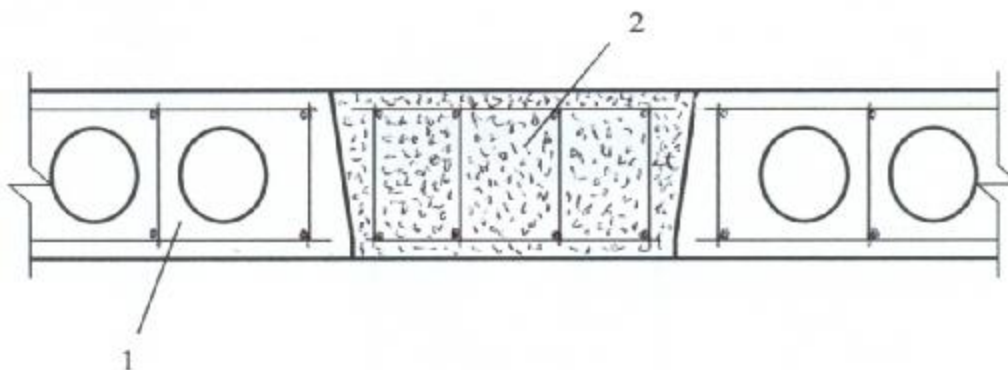
Рис. 4. Сборно-монолитное перекрытие:
