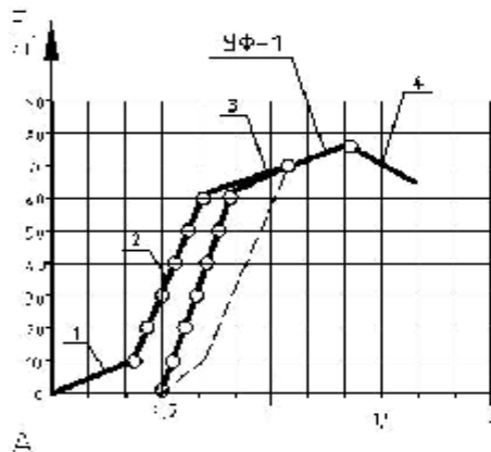
Рис. 3. Графики зависимости деформаций смещения стержневых элементов в узловых соединениях структурной системы УФ от сжимающих нагрузок: А – Узловое соединение 1; Б – Узловые соединения 2, 3; 1, 2, 3, 4 – стадии работы узлового соединения
