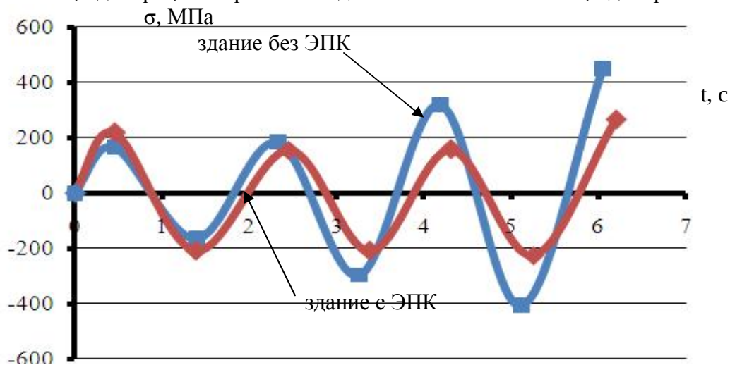
Рис. 2. Изменение напряженного состояния в колонне 1-го этажа
