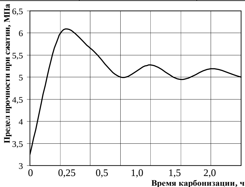
Рис. 3. Зависимость изменения прочности на сжатие опытных образцов из мраморовидного известняка от времени обработки их уголекислым газом
