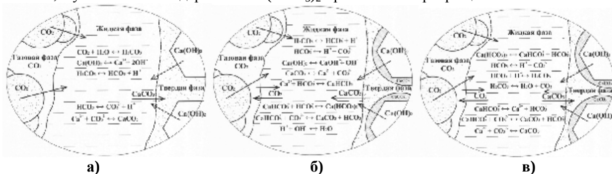
Рис. 2. Механизм образования вторичного карбоната кальция в системе « \text{Ca(OH)}_2 - \text{H}_2\text{O} - \text{CO}_2 »: а) стадия образования карбоната кальция; б) стадия растворения \text{CaCO}_3 и образование в системе \text{Ca(HCO}_3)_2 ; в) стадия превращения \text{Ca(HCO}_3)_2 в \text{CaCO}_3
