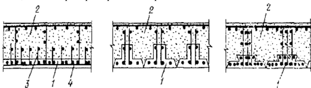
Рис. 3. Сборно-монолитные железобетонные панели под большие нагрузки (до 500 кН/м 2 ):
