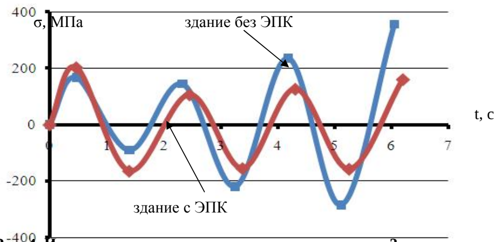
Рис. 4. Изменение напряженного состояния в колонне 3-го этажа
