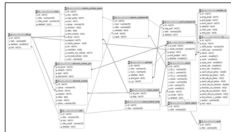
Рисунок 2. Физическая модель базы данных учета успеваемости обучающихся
