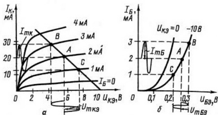
Рисунок 2. Графики напряжений и токов в транзисторном усилителе, работающем в режиме А
