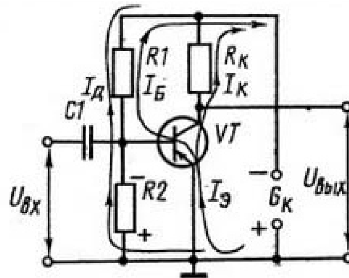
Рисунок 3. Схема транзисторного усилителя с фиксированным напряжением базы
