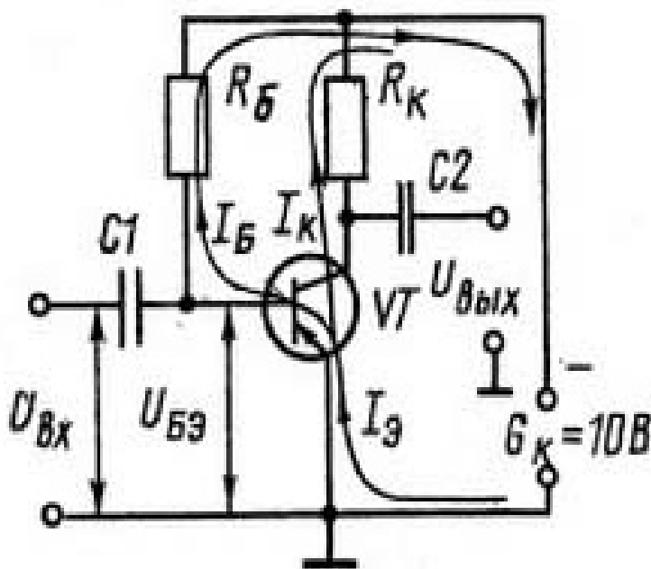
Рисунок 1. Схема транзисторного усилителя с фиксированным током базы
