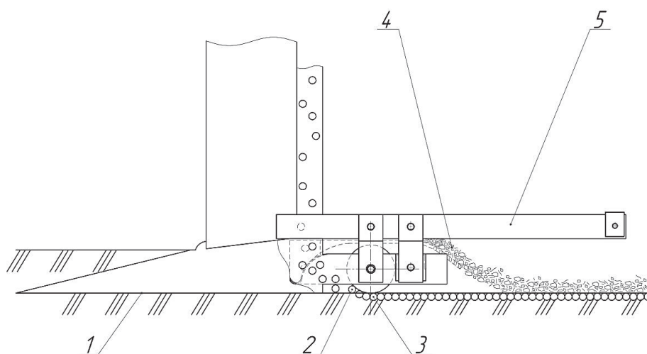
Рис. 1. Технологическая схема посева с прикатыванием на уровне залегания семян: 1 – образование равномерно-уплотненного семенного ложа путем подрезания почвы лапой сошника, 2 – распределение и укладка семян, 3 – место непосредственного процесса обеспечения качественного контакта семян с почвой, 4 – перемещение подрезанного слоя
