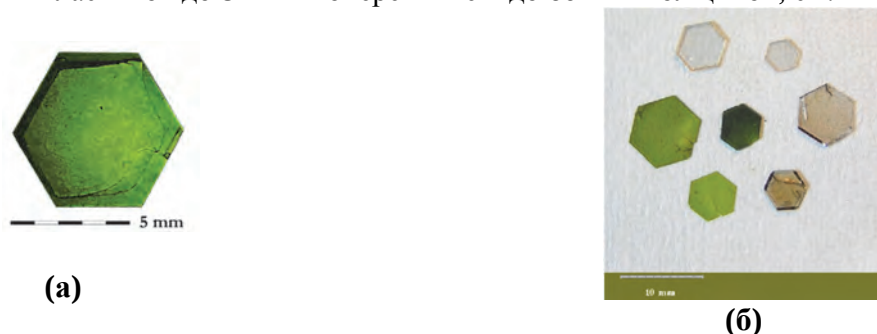
Рис. 1. Синтезированные монокристаллы (а) \text{FeBO}_3 и (б) \text{Fe}_{1-x}\text{Ga}_x\text{BO}_3 с различными x .
