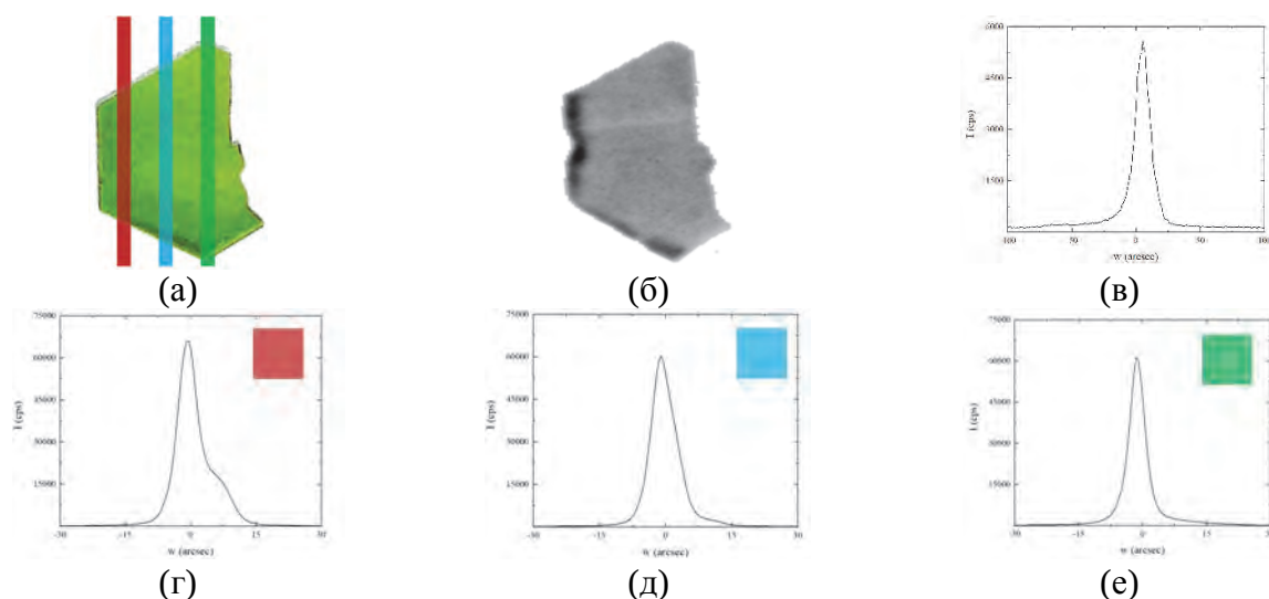
Рисунок 1. Монокристалл \text{FeBO}_3 : оптическая микроскопия (а), рентгеновская топограмма (б) и кривые качания, снятые интегрально (в) и локально (г,д,е) (рефлекс (0012) ).
