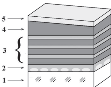
Рис. 1 – Схема структуры GGG/Au NP /M1/( \text{SiO}_2 /M1) 3 / \text{SiO}_2 (клин)/Au
