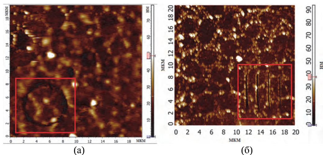
Рис. 1. Результаты проведения литографии на покрытии Си: а – векторная литография и б – растровая (полоски) литография.
