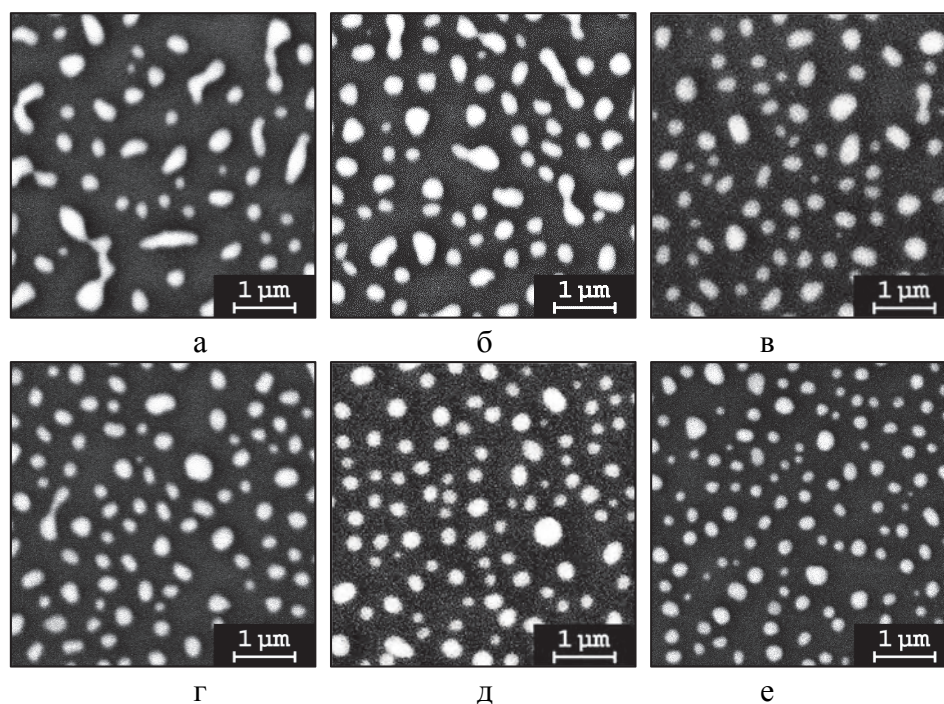
Рис. 1. Морфология поверхности плёнки Au/GGG ( h_{eff} = 10 нм) после ТАГ при 680°C: а – 1 мин, б – 2 мин, в – 5 мин, г – 10 мин, д – 30 мин, е – 60 мин.
