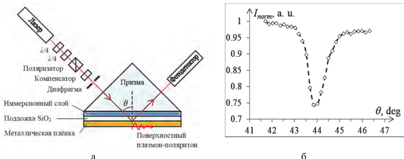
Рис.1 Зависимость интенсивности отраженного света от поверхности пленки от угла падения светового пучка.
