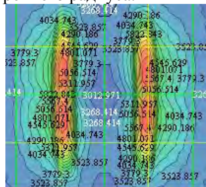
Рис 3. \sigma_{33} при t^1=0.49
