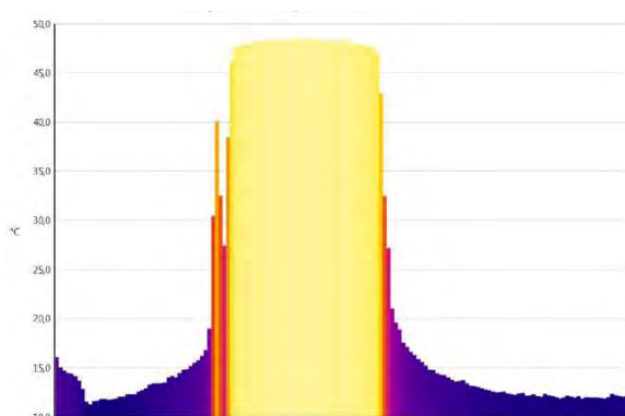
Рис. 2. Термограмма поверхности внешней ограждающей конструкции Минимум – 11 °С. Максимум – 47,8 °С. Среднее значение – 20,8 °С
