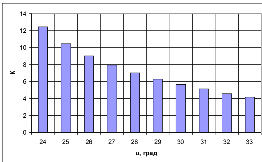
Рисунок 7 – Зависимость коэффициента концентрации от угла наклона второй и третьей фацеты
