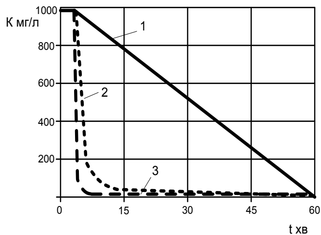
Рис.2. Изменение концентраций загрязнений в период процесса водоочистки технологии реагентной коагуляции. 3 - изменение концентрации несоагулированных частиц дисперсных примесей, 2 - изменение концентрации дисперсных примесей в очищаемой воде, при осаждении скоагулированных частиц, 1 - изменение концентрации очищаемой воды, в водоприемнике, \tau - настоящее время, мин.
