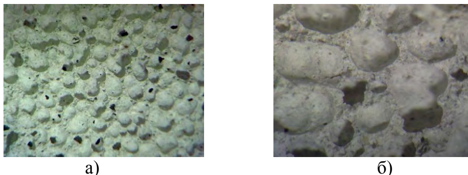
Рис. 2. Структура газобетона плотностью 600 кг/м 3 на основе цементно-известкового вяжущего и мелкодисперсного мраморовидного известняка, увеличение: а – \times 8 ; б – \times 28
