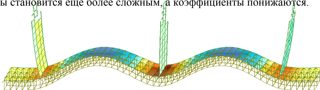
Рис. 7. Фрагмент деформированной схемы плиты
