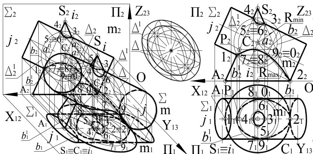
Рис. 6. Результаты построения линии пересечения поверхностей вращения.
