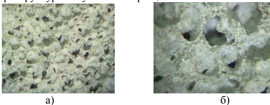
Рис. 1. Структура газобетона плотностью 600 кг/м 3 на основе цемента и песка, увеличение: а – × 8; б – × 28
