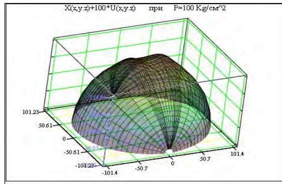
Вид половины сферы в деформированном состоянии. t^1=0.01
