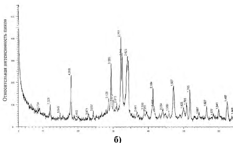
Рис. 7. Рентгенограмма продуктов гидратации портландцементного камня в возрасте 28 сут: а – без дисперсных волокон; б – с базальтовым волокном
