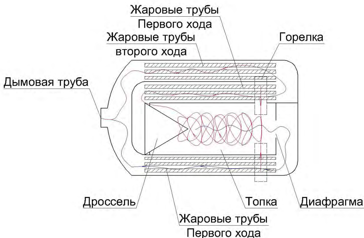
Рис. 7 Предложенная модель топки жаротрубного котла мощностью от 100 до 300 кВт.
