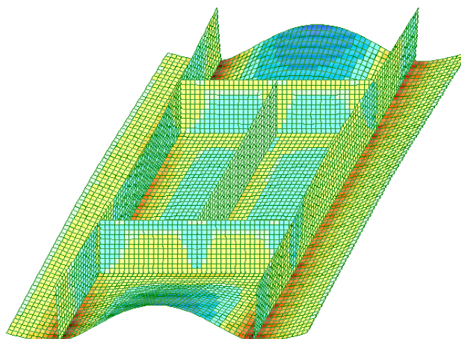
Рис.2. Изополя напряжений в плите базы колонны
