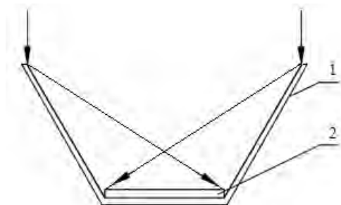
Рисунок 2 – Факетный концентратор, состоящий из двух плоских отражателей 1- плоский отражатель (зеркало); 2 – приемник солнечного излучения
