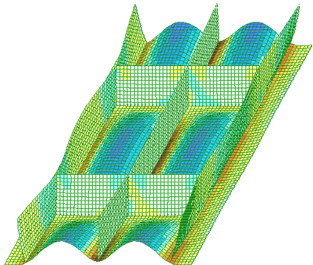
Рис. 5. Деформированная схема плиты с установленными ребрами
