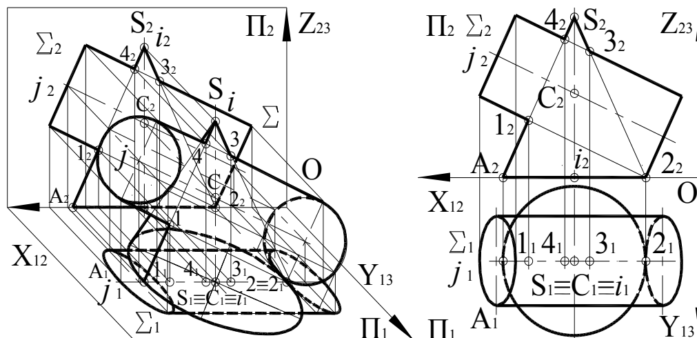
Рис. 5. Трехмерные и двухмерные модели исходных геометрических образов конуса и цилиндра.
