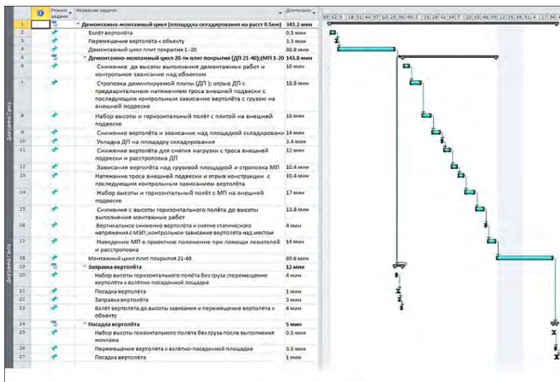
Рисунок 3 - Фрагмент модели МДР с совмещенными площадками
