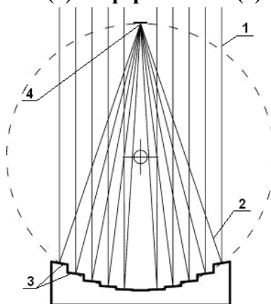
Рисунок 3 – Цилиндрический (а) и сферический (б) факетные концентраторы
