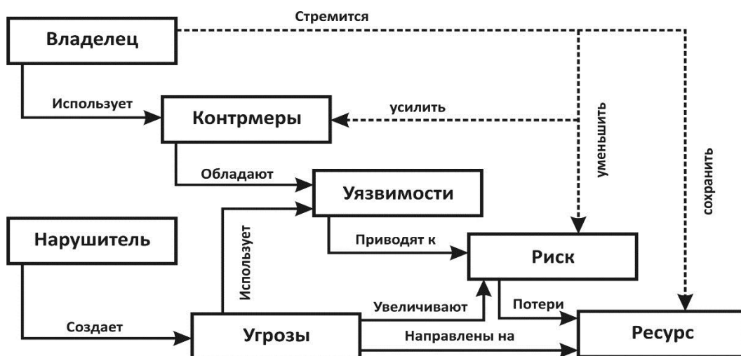
Рис.1. Модель построения корпоративной системы защиты информации
