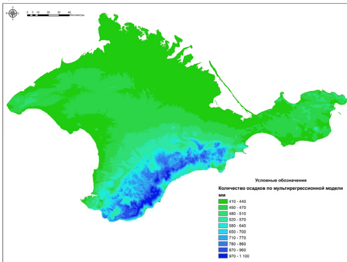
Рис.1. Результаты визуализации мульти-регрессионной модели осадков для Крыма
