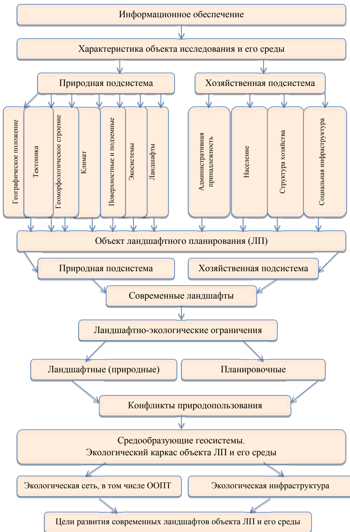
Рис. 1. Схема методики ландшафтного планирования территории Большой Ялты
