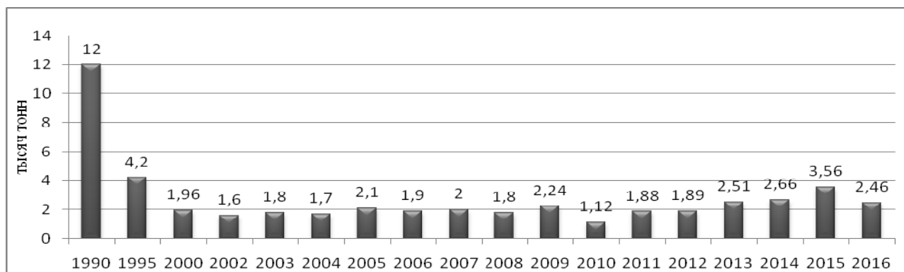
Рис. 1. Динамика выбросов загрязняющих веществ в атмосферный воздух стационарными источниками в городе Симферополь
