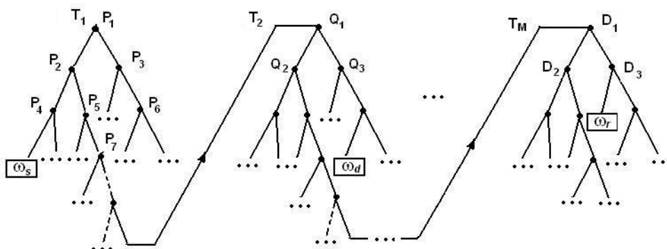
Рис. 1. Схема взаимодействия ансамбля решающих деревьев
