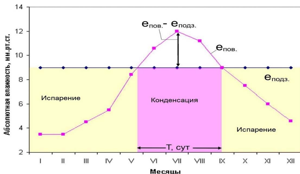
Рис. 1. Определение продолжительности и интенсивности конденсации в водосборе Петровского источника
