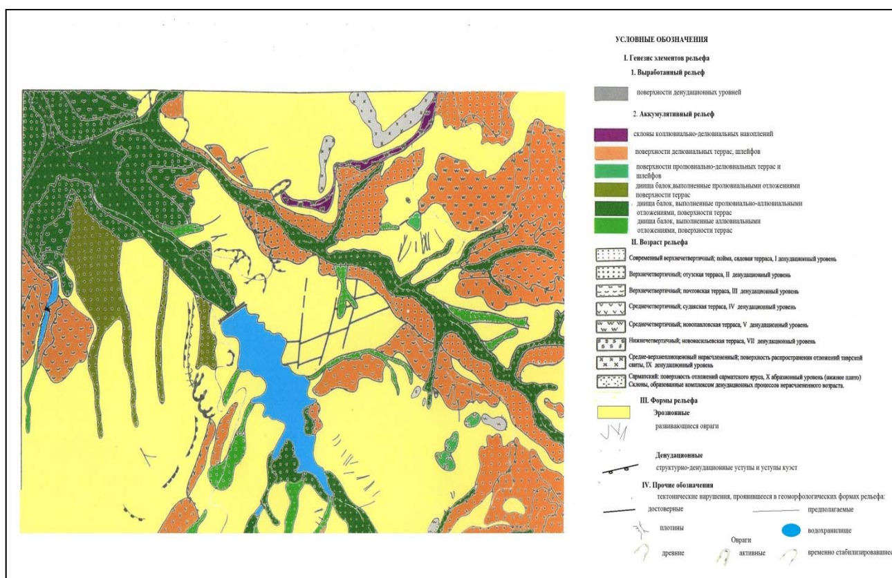
Рис.1. Схематическая геоморфологическая карта долины реки Малый Салгир
