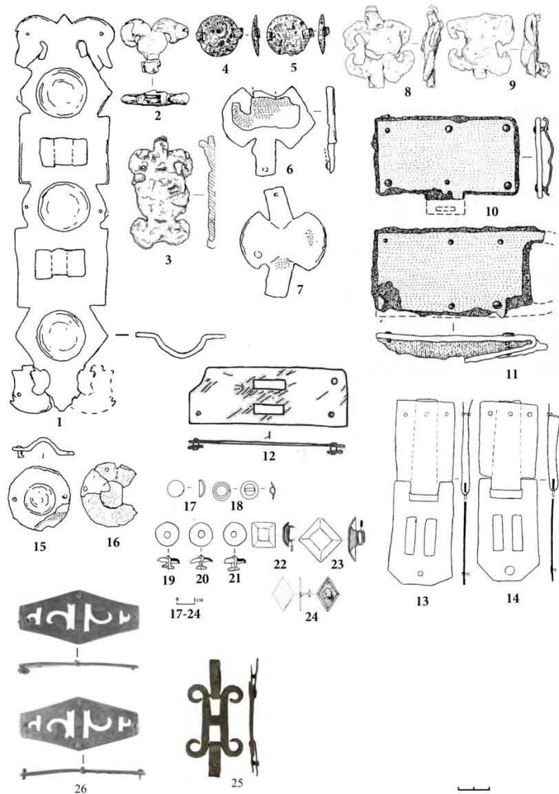
Рис. 28. Налобные и накладные бляхи: 1,6-7, 15-18 – погребение у ворот Неаполя скифского (по Зайцев, Мордвинцева, 2007); 2 – могила №1 Опушки (по Храпунов, 2007); 3 – могила №355 Нейзац (По Храпунов, 2015); 4,5 – могила №223 Бельбек IV (по Ахмедов, Гущина, Журавлев, 2001); 8-9 – северный подбой могилы №374 Нейзац (по Храпунов, 2015); 10-11 – погребение у хут. Оланешты (Курчатов, Бабулич, 2003); 12 – курган 9 у с. Нагорное (Гудкова, Фокеев, 1984); 13-14 – склеп №17 Нейзац (по Храпунов, Мульд, 2004); 19-21 – могила №300 Нейзац (по Храпунов, 2011a); 22-23 – могила №306 Нейзац по Храпунов, 2011); 24- могила №3 Дружное (по Храпунов, 2002); 25 - могила 319 могильника Фронтное 3 (по Гавритухин, Свиридов, Язиков, 2020); 26 - погребение 58 могильника Киль-Дере (по Дорошко, Свиридов, Язиков, 2022). 1-11,15,16 – железо, позолота; 12,19-23 – серебро; 13-14, 25-26 – бронза;17-18, золото; 24 – бронза, серебро.
