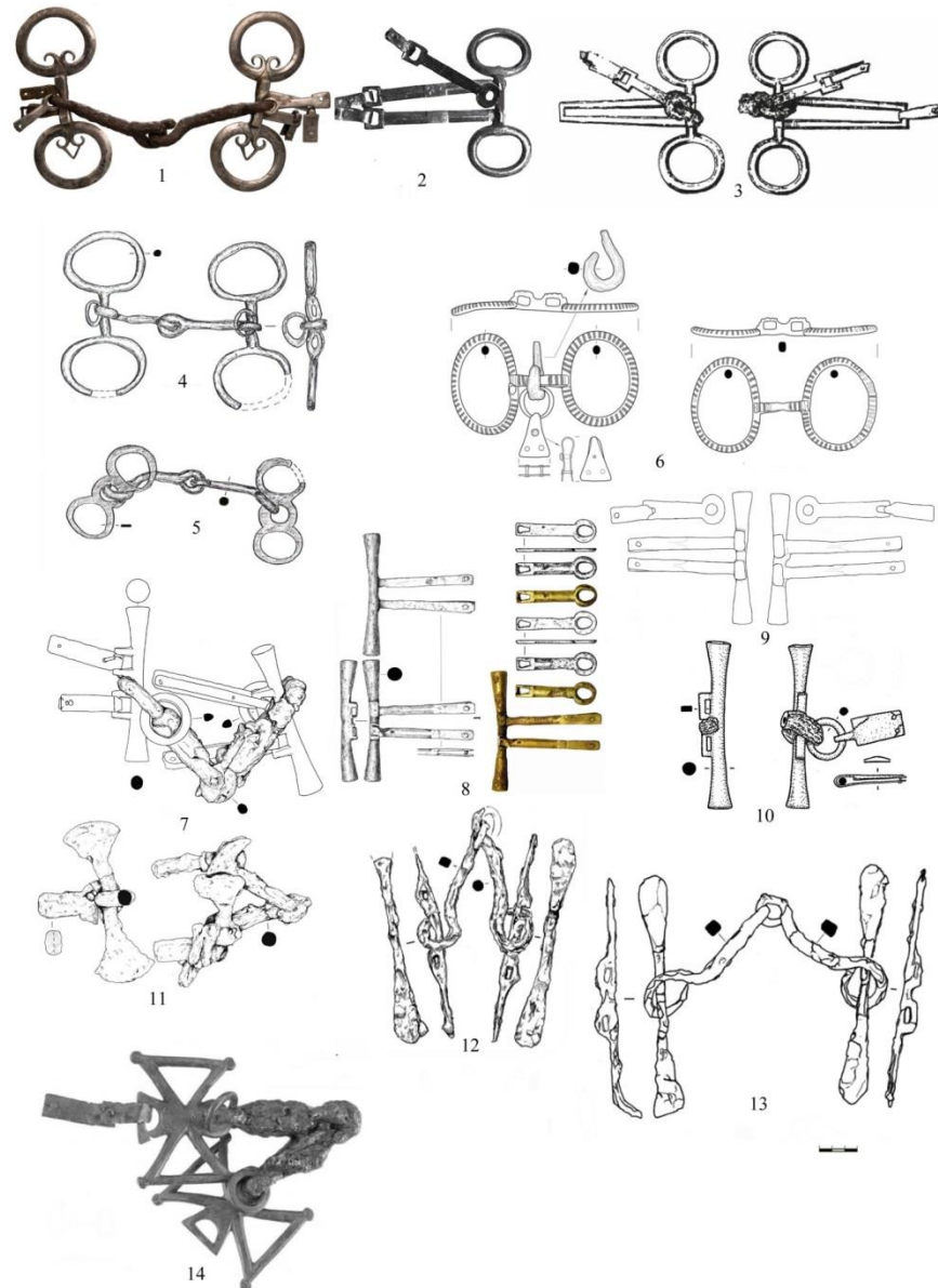
Рис. 21. Тип III. Стержневидные: 1 – погребение 1, курган 25, могильник Валовый I (по Трейстер, 2020); 2 – погребение лошади на некрополе Херсонеса (по Симоненко, 2013); 3 – псалии из грунтового некрополя Пантикапея (по фон Штерн, 1898); 4,5 - псалии из грунтового могильнике городища №1 у хутора Ленина (по Лимберис, Марченко, 2022); 6 – псалии из кургана 12 Никольского могильника (по Лимберис, Марченко, 2022); 7 – псалии из могилы №183 могильника Нейзац (по Антипенко, 2015); 8 – псалии из склепа №4 (77) Чернореченского могильника (по Антипенко и др., 2021); 9 - случайная находка у с. Червоный Чабан Херсонской области (по Антипенко и др., 2021); 10 - псалии из Горгиппии (по Новичихин, 2011); 11 – могила №374 Нейзац (по Храпунов, 2015); 12, 13 – конские погребения могильника Опушки (по Храпунов, Шабанов, 2021); 14 - погребение 58 могильника Киль-Дере (по Дорошко, Свиридов, Языков, 2022).
