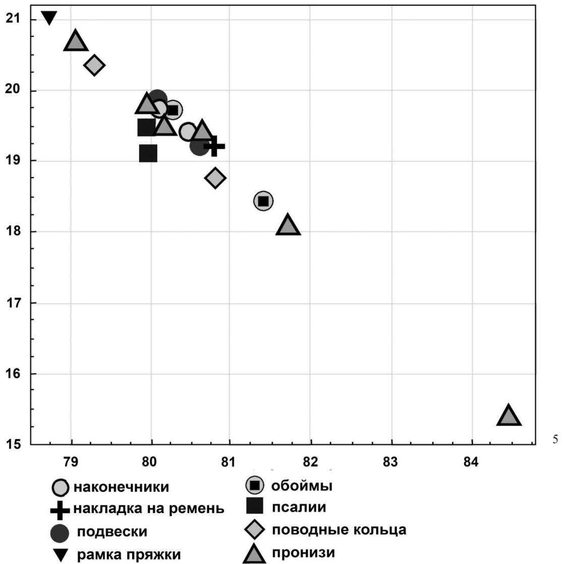
Рис. 37. 1-4 – конская амуниция из некрополя Горгиппии, 5 – график распределения основных компонентов сплава в деталях конской амуниции из склепа 4 (77) Чернореченского могильника.
