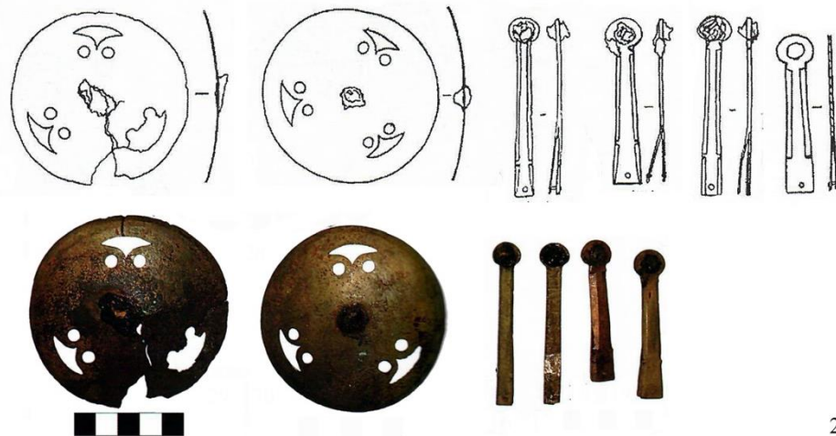
Рис. 18. 1 – Фото и прорисовка псалий из погребения 1 кургана 3 курганной группы «Большевик II» (по Безуглов, Нидзельницкая, 2020); 2 – фото и прорисовка псалий из погребения 73 некрополя Кобякова городища (по Ларенок, 2003).
