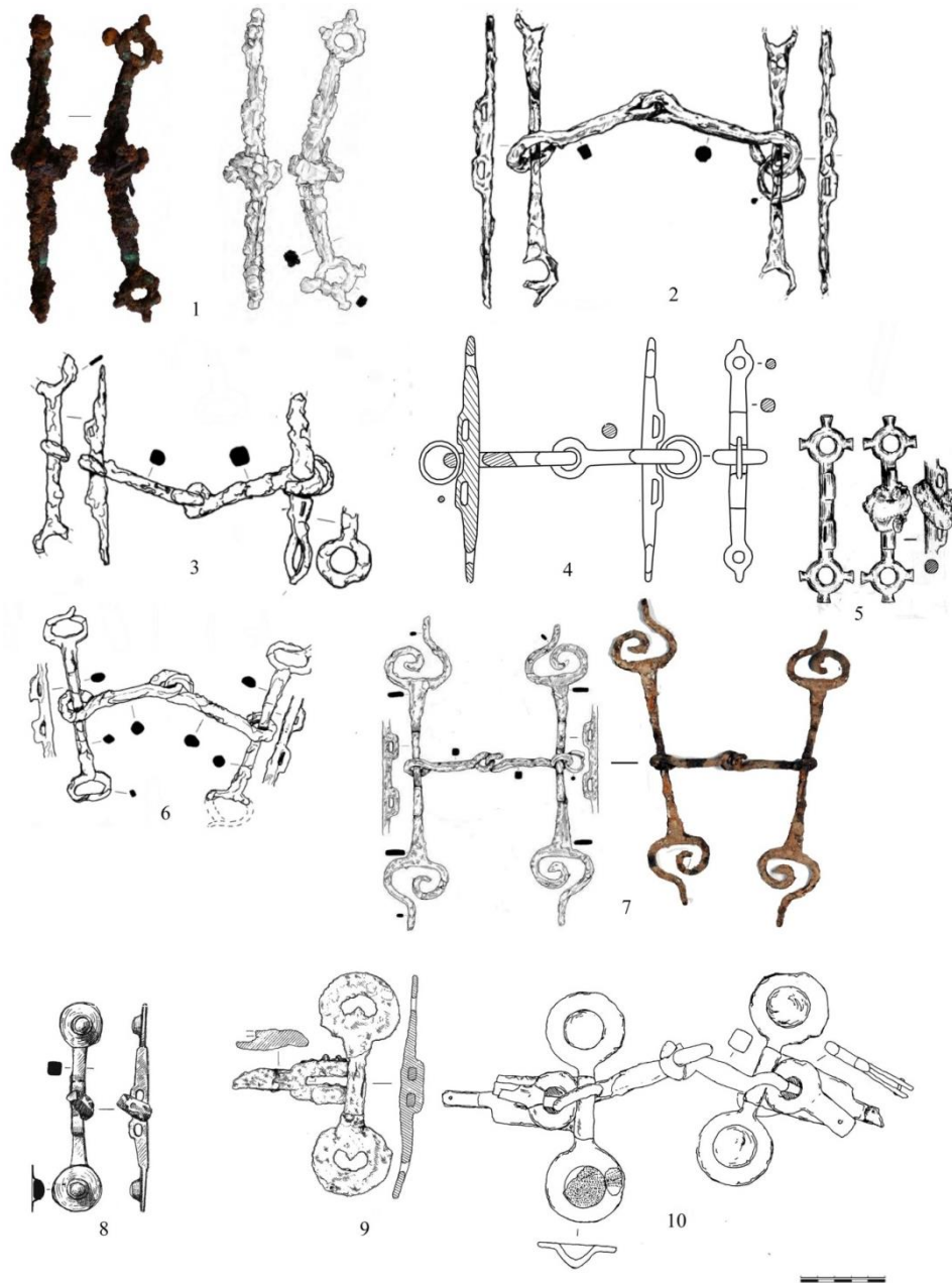
Рис. 20. Тип III. Стержневидные: 1 – фото и прорисовка псалий из склепа №777 могильника Усть-Альма (по Пуздровский, Труфанов, 2017); 2,3 - конские захоронения могильника Опушки (по Храпунов, Шабанов, 2021); 4 – погребение 1, кургана 1 могильника Октябрьский V (по Мыськов, Кияшко, Скрипкин, 1999); 5 – курган 43 у ст. Усть-Лабинская (по Гушина, Засецкая, 1994); 6 – могила №181 могильника Опушки (по Храпунов, Шабанов, 2021); 7 – прорисовка и фото псалий из могилы №86 некрополя Левадки (по Мульд, 2009); 8 – конская могила №3/1997 могильника Усть-Альма (по Пуздровский, 2007); 9 – могила №355 могильника Нейзац (по Храпунов, 2015); 10 – погребение на городище Неаполь скифский (по Зайцев, Мордвинцева, 2007).
