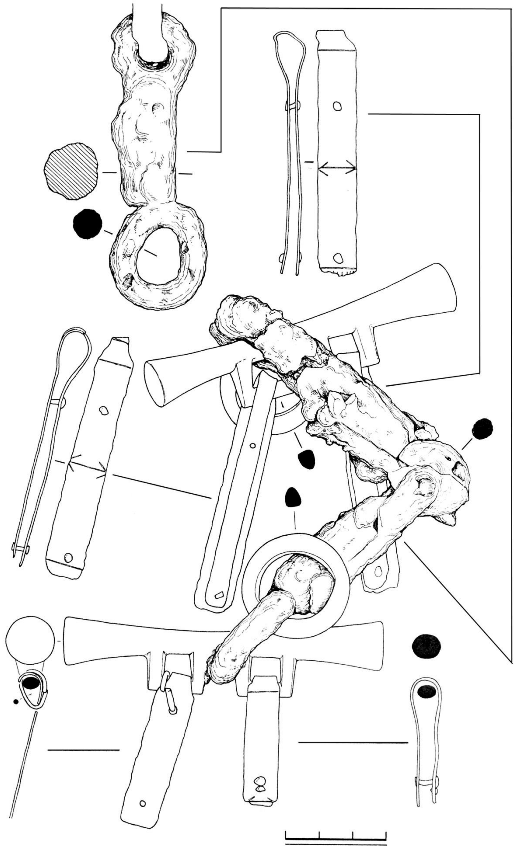
Рис. 38. Удила и псалии из могилы №183 могильника Нейзац.
